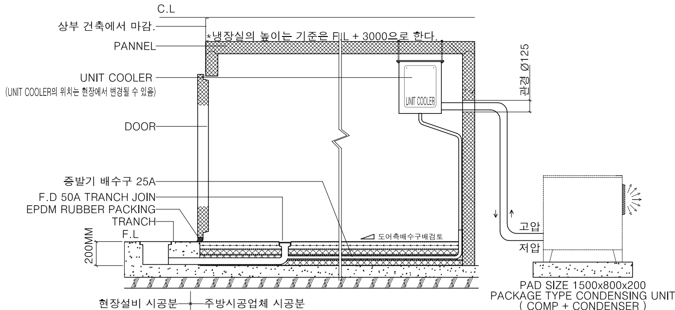
조립식냉장실/냉동실 배수배관상세도
