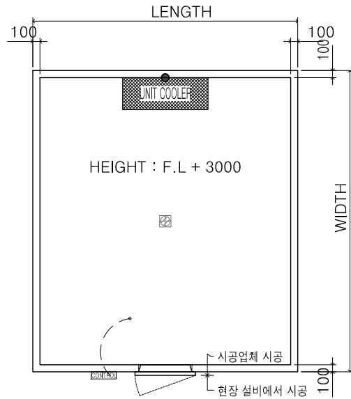
조립식냉동/장실 평면도
