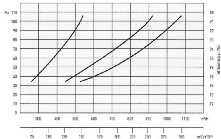
<풍압, 정압, 스크린 성능 분석표>
