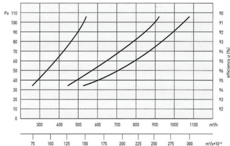
<풍압, 정압, 스크린 성능 분석표>
